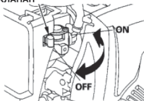
ТОПЛИВНЫЙ КЛАПАН
